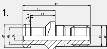
1. ISO 7388-3 Forma AD con foro passante/Form AD with drill through (Norma precedente/previous norm DIN 69872 Form A)
