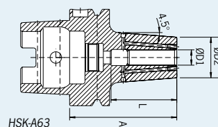
HSK-A63
