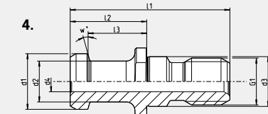
4. JIS B 6339 con foro passante/with drill through
